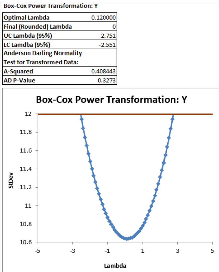
Fig. 4.49 Box-Cox output
