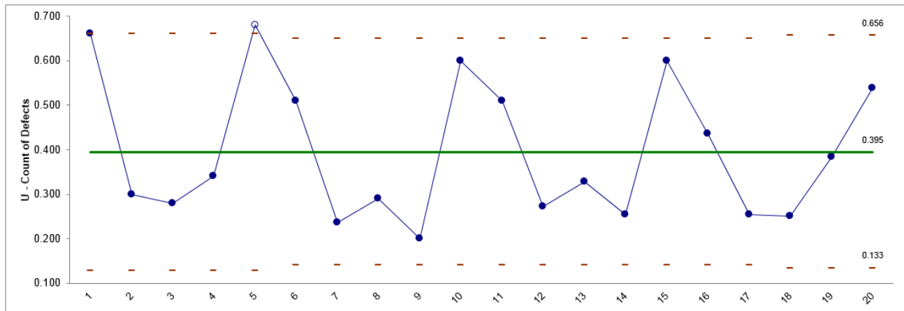
Fig. 5.12 U-Chart output
