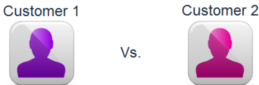
Fig. 3.67 Mann-Whitney Test
